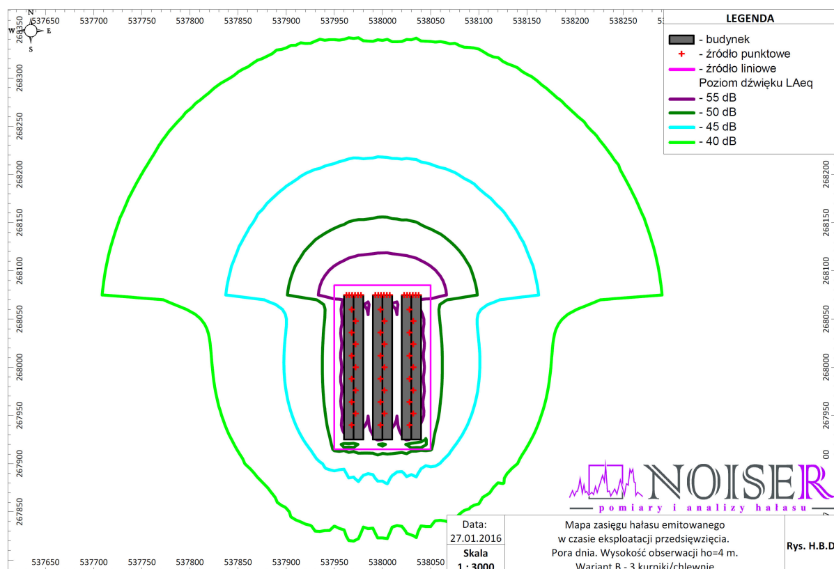
Ryc. 31. Orientacyjny zarys obszaru przekroczeń dopuszczalnych natężeń hałasu w środowisku w wariacie trzech obiektów obok siebie.
