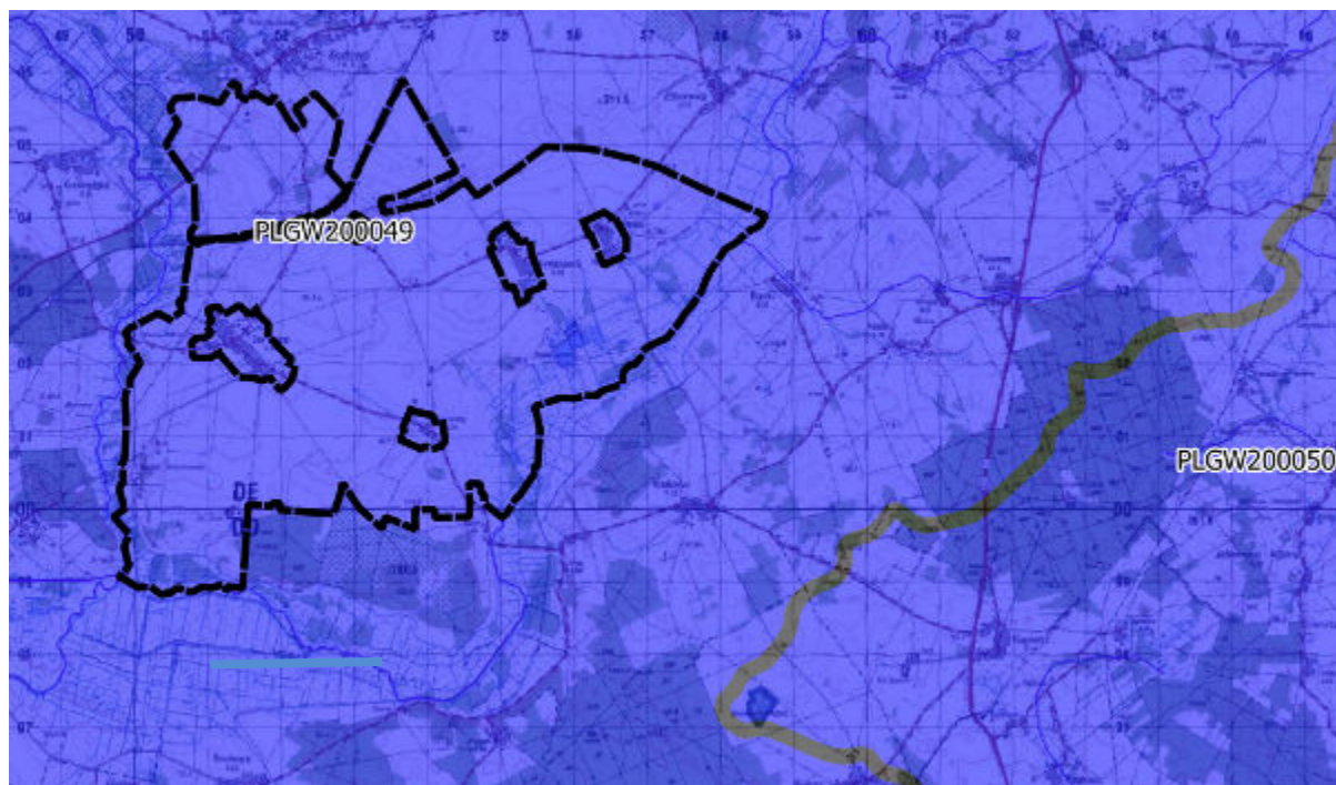
Ryc.20. Jednolite części wód podziemnych (JCWPd) na terenie opracowania (podkreślone niebieską linią). Obszar opracowania – czerwona obwiednia. Źródło: http://geoportal.kzgw.gov.pl/imap/
