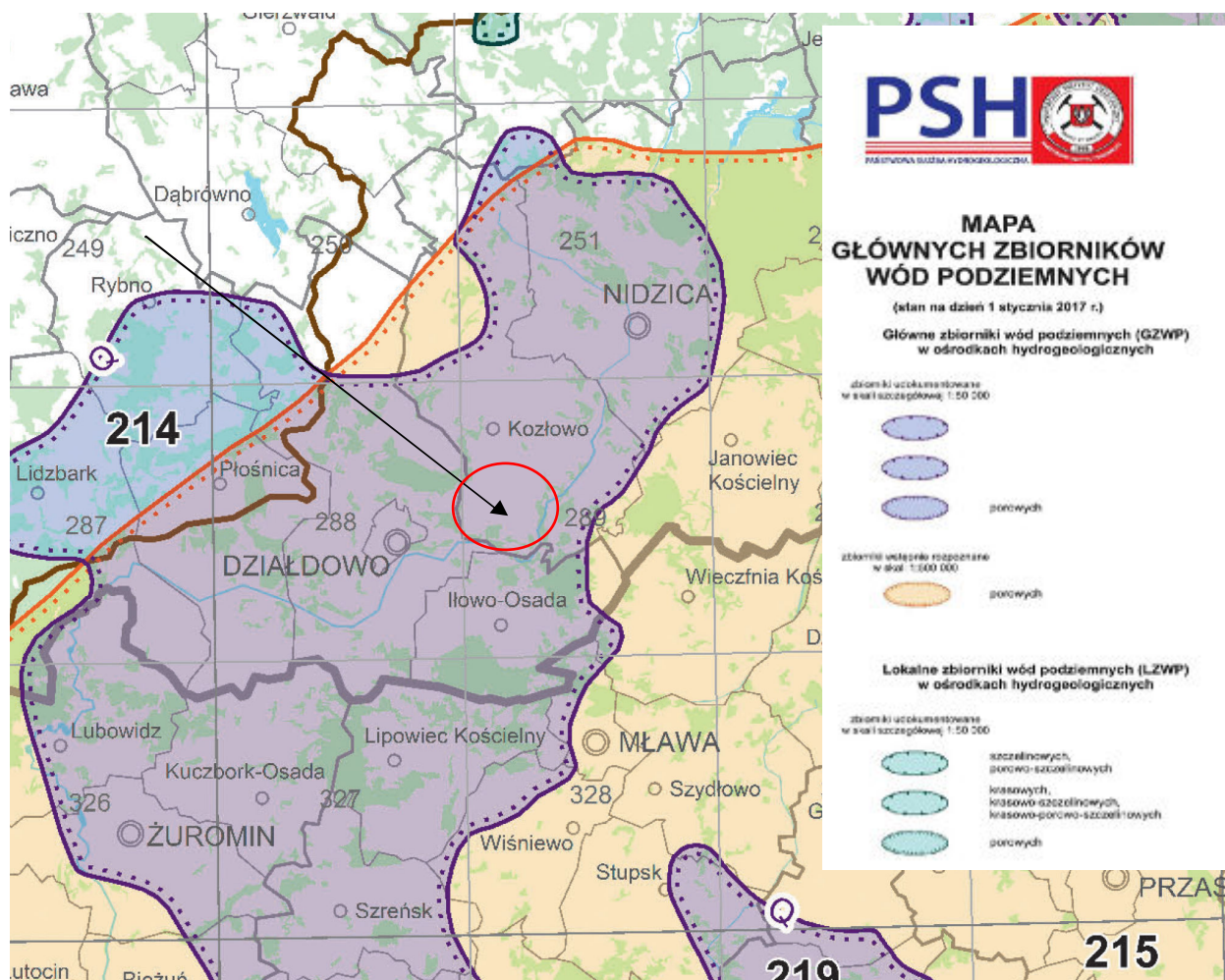
Ryc.18. Mapa GZWP na terenie gminy Kozłowo – czerwony okrąg i strzałka wskazuje orientacyjnie położenie obszaru opracowania.
