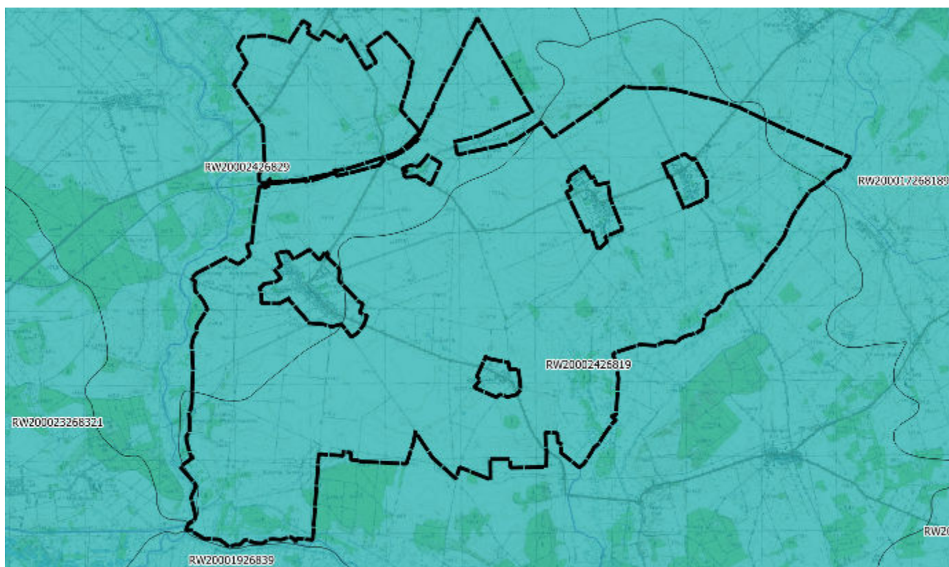
Ryc.19. Jednolite części wód powierzchniowych (JCWPw) na terenie granic opracowania. Źródło: http://geoportal.kzgw.gov.pl/imap/
