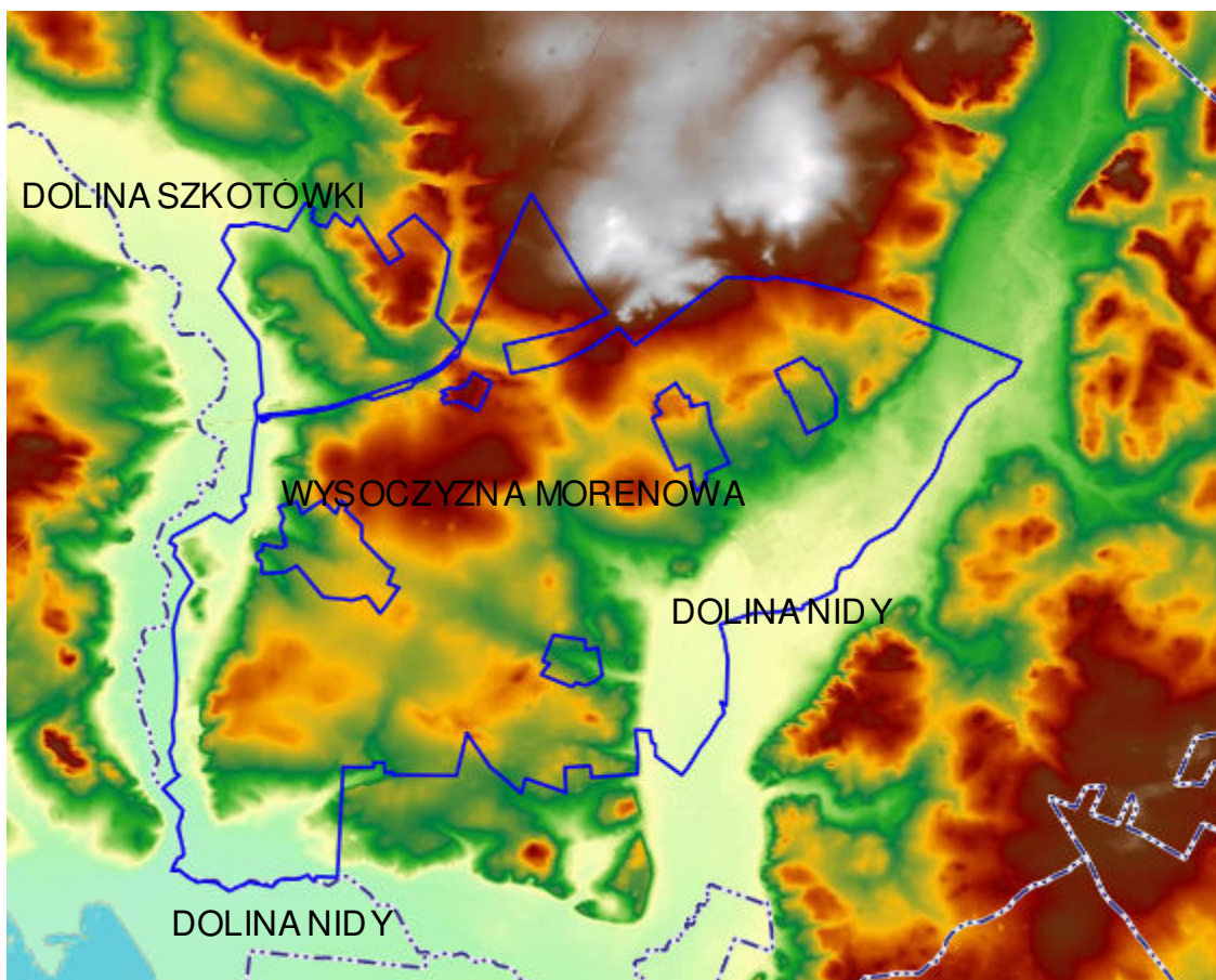
Ryc. 15. Ukształtowanie terenu opracowania. Źródło: www.geoportal.gov.pl
