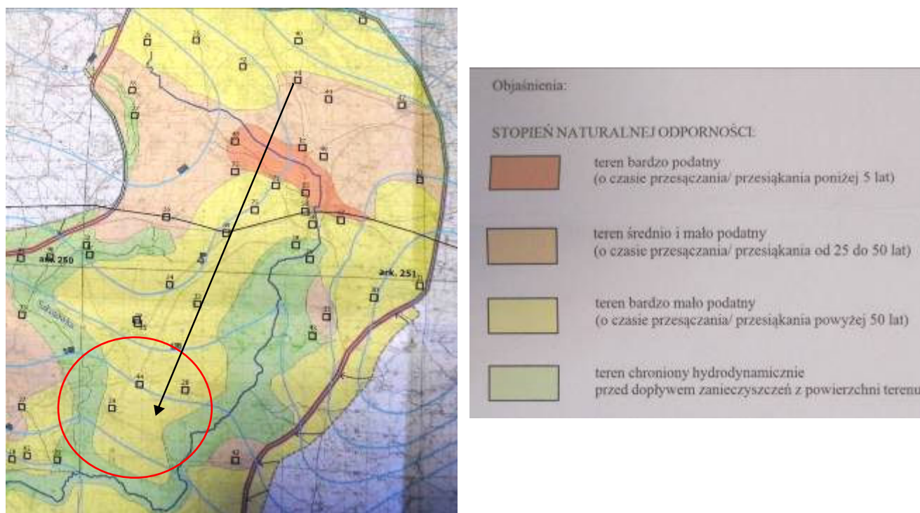
Ryc.18a. Mapa GZWP zawierająca dane na temat naturalnego stopnia odporności na przenikanie zanieczyszczeń do wód zbiornika – fragment mapy z Dokumentacji Hydrogeologicznej zbiornika 214 Działdowo opracowanego przez POLGEOL S.A. - J. Niewiarowicz, J. Kapuściński, Warszawa, 2013. Czerwony okrąg i strzałka wskazuje orientacyjnie położenie obszaru opracowania.
