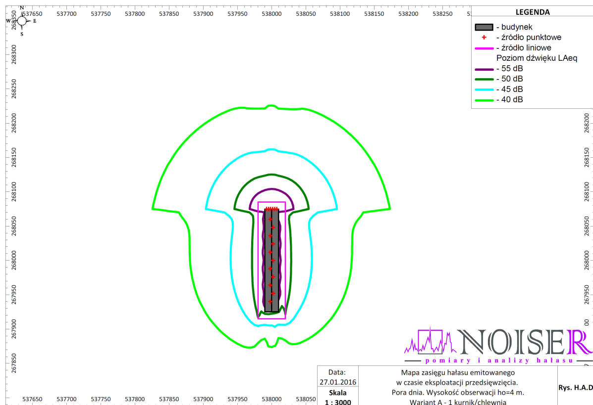
Ryc. 30. Orientacyjny zarys obszaru przekroczeń dopuszczalnych natężeń hałasu w środowisku w wariantach A i B pojedynczego obiektu.
